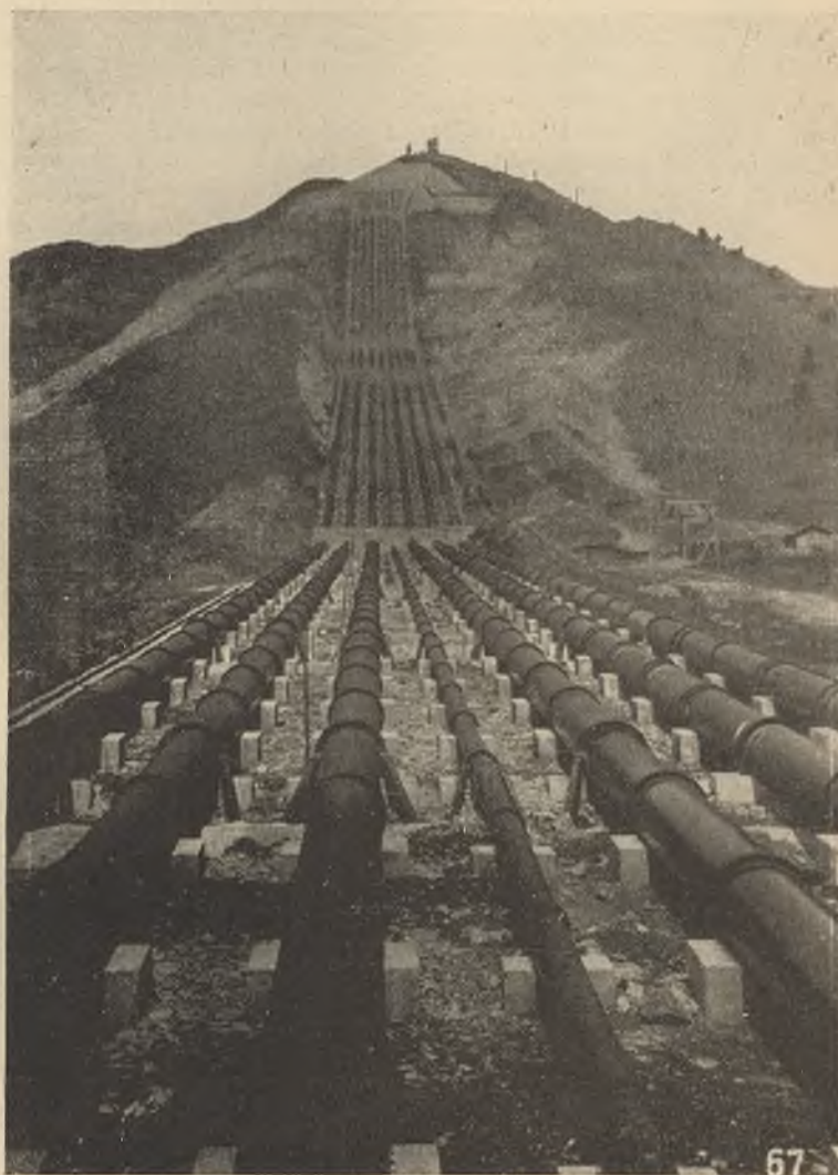
Stacja hydroelektryczna, Kinugawa w Japonii. Rurociągi dostarczyła i zmontowała Sp. Akc. „Ferrum“, Katowice.
