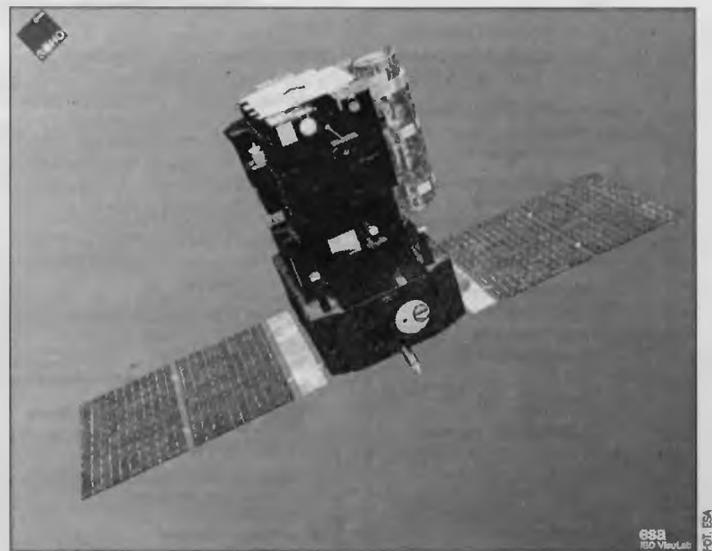
SOHO – najstarsze kosmiczne obserwatorium Słońca.
