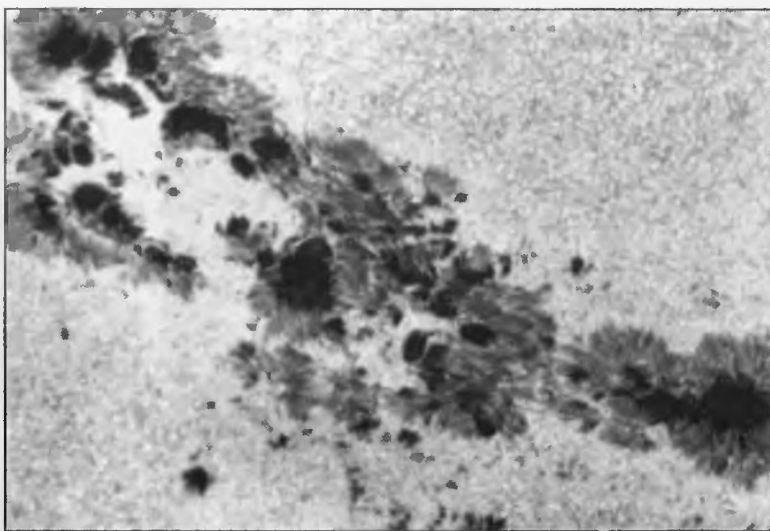
Plamy słoneczne – potężne zawirowania w polu magnetycznym.
