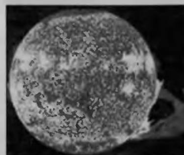
Chromosfera słoneczna z potężną protuberancją.
