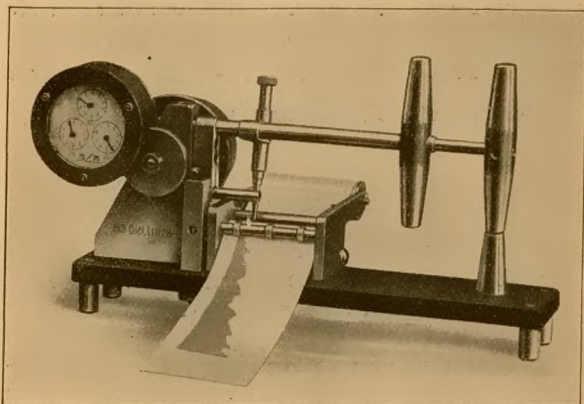
Nr. 259. Registrler-Handergometer nach Prof. Dr. Klemm
