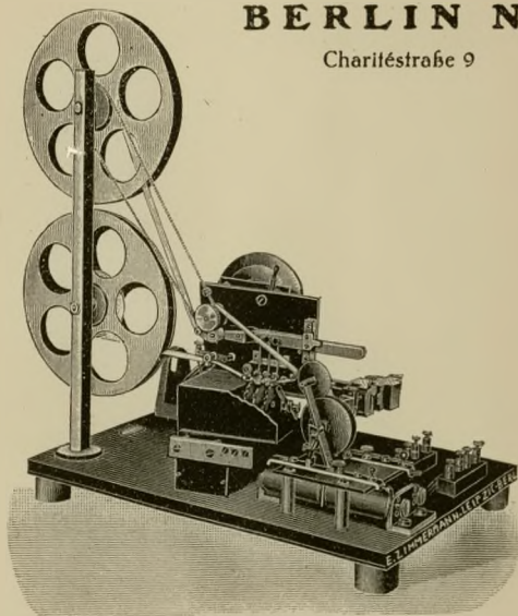
Zählender Chronograph nach Lewin
