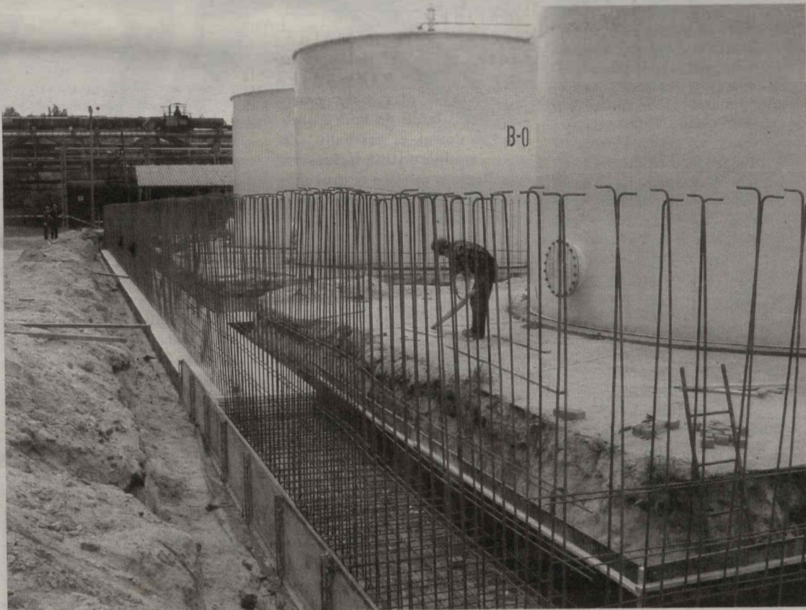
Ściany nowych tac ochronnych wychodzą z ziemi
