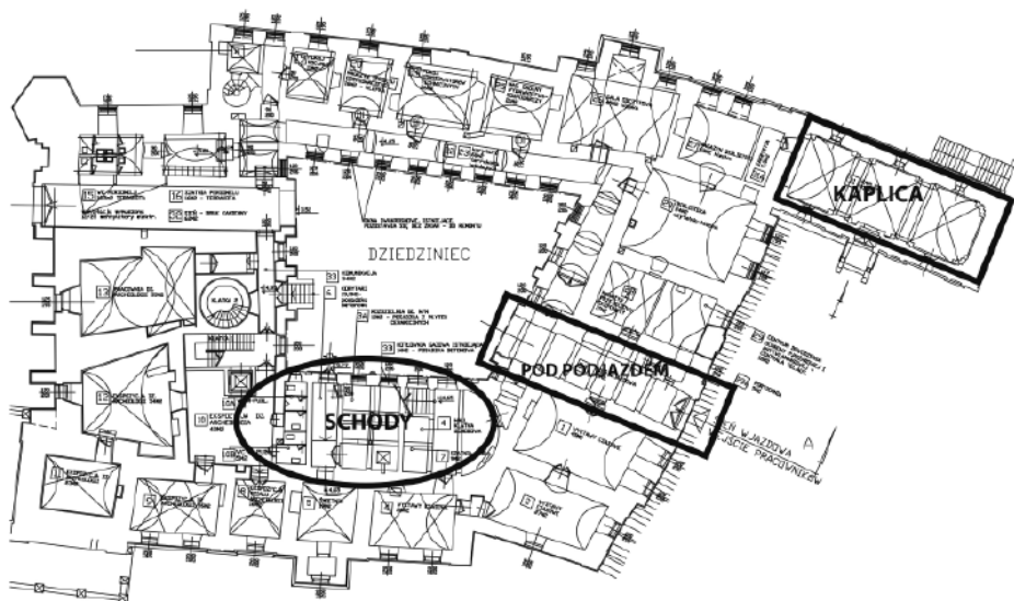
Współczesny plan pomieszczeń zamku książąt Sułkowskich w Bielsku-Białej – parter Źródło: Muzeum Historyczne w Bielsku-Białej.
