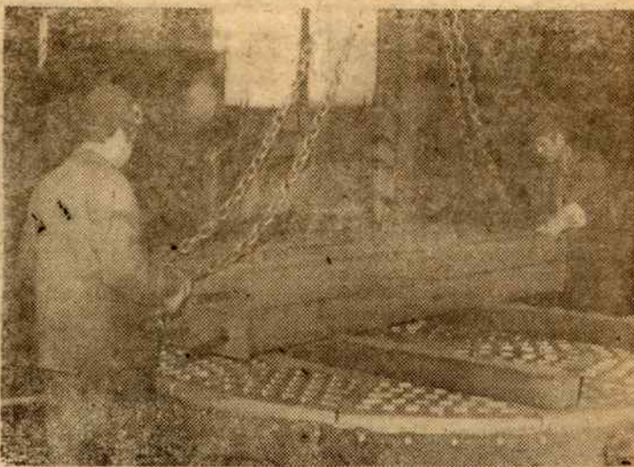
Wycinanie rur żebrowych ze śrutownicy. Na zdj. R. Zbylut i Cz. Tomaszko.
