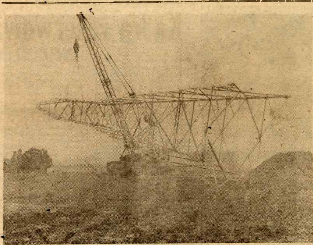
ZWSE — budowa linii przesyłowej.
