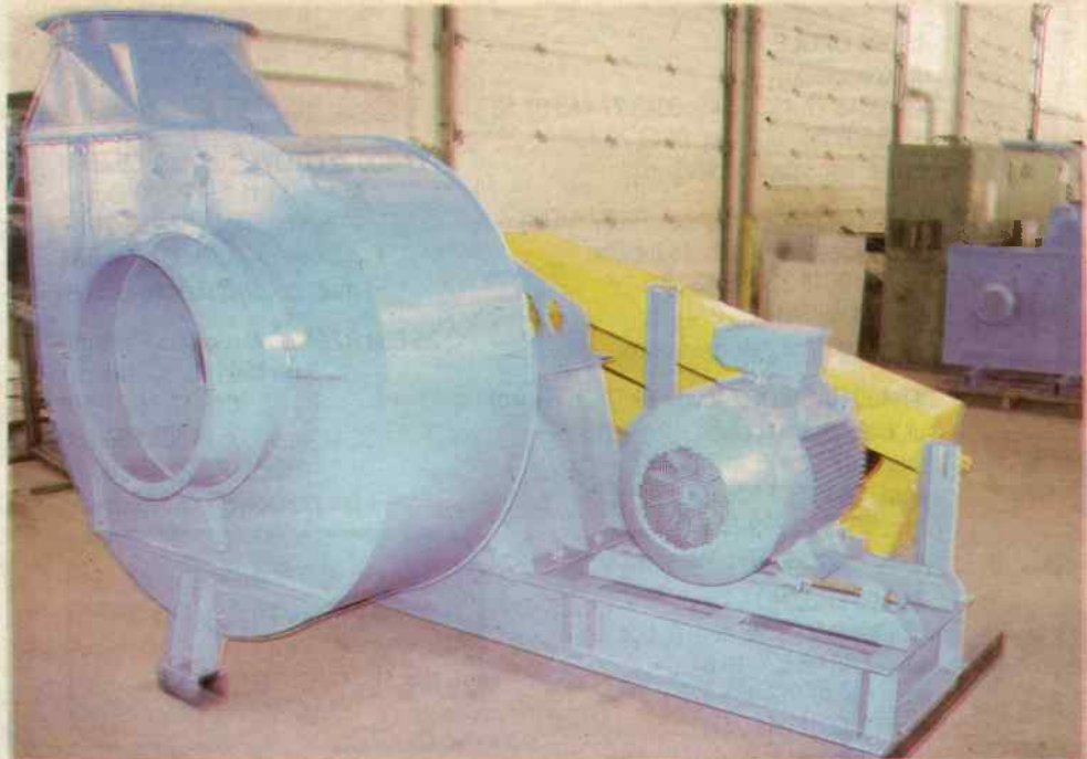
Tak wyglądają wentylatory produkowane w NETECS-ie. To jeden z największych o mocy 75 kilowatów.
