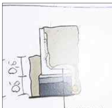
Grunt zostanie ustabilizowany dzięki betonowemu elementowi w kształcie litery L
