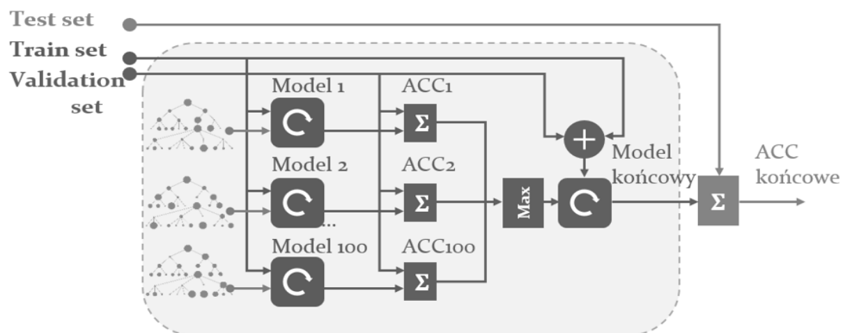
Rysunek 9.15: Schemat zagnieżdżonej walidacji krzyżowej.
