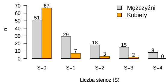
(b) HOLTER_II .
