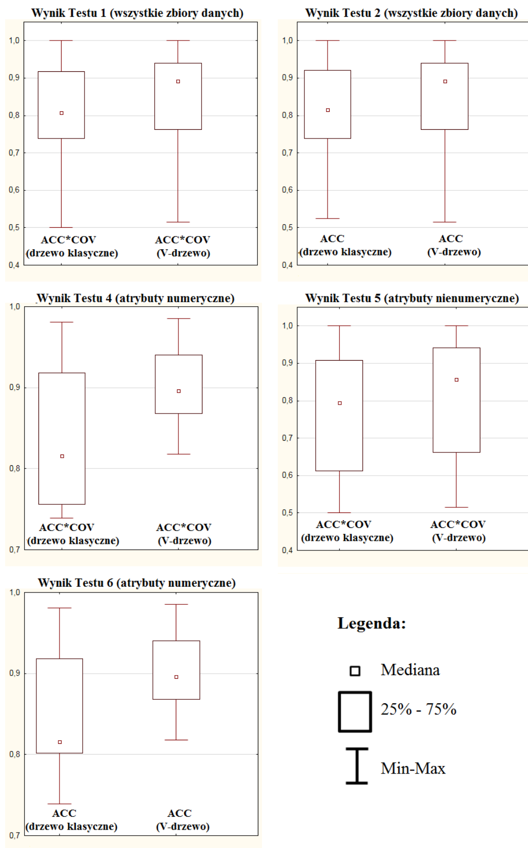
Tablica 9.33: Wykresy pudełkowe testów z poziomem istotności poniżej 0.05.
