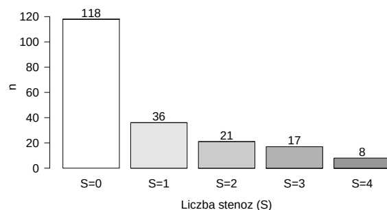
(b) HOLTER_II .
