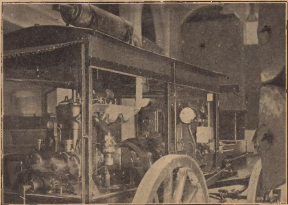
Wóz — świetlny, agregat benzynowy. służący jako własna ruchoma elektrownia na plenerach. „Diana-Film“ w Poznaniu.
