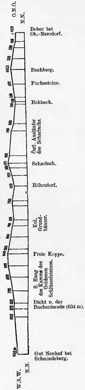
Querprofil durch das mittlere Drittel des Landeshuter Kammes und seiner Nebenketten. Längen- und Höhenmaßstab 1 : 100.000.
