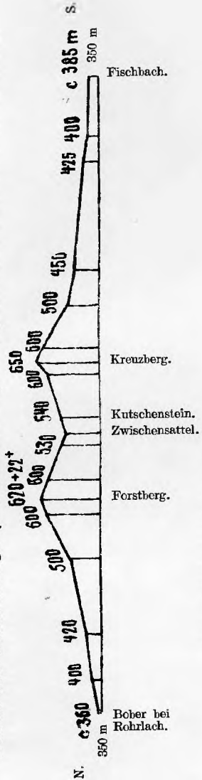
Profil der Falkenberge (Ansicht von W.). Längen- und Höhenmaßstab 1 : 25.000.
