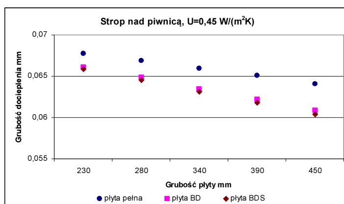
Rys. 6. Grubość warstwy docieplenia styropianem dla stropu nad piwnicą
