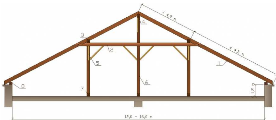
Rys. 4. Konstrukcja dachu płatwiowo - kleszczowa z płatwią kalenicową i płatwiami pośrednimi: 1- krokiew, 2 - kleszcze, 3 - płatew pośrednia, 4 - płatew kalenicowa, 5 - miecz, 6 - słup, 7 - płatew podwalinowa, 8 - murlata [5]
