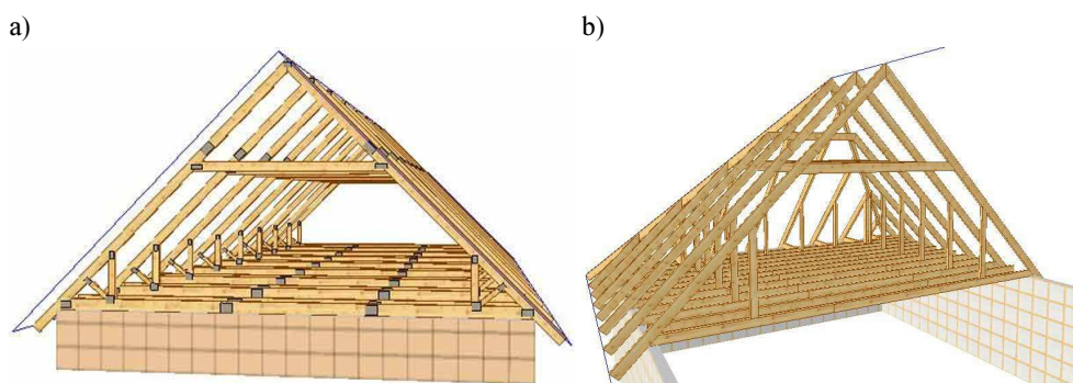
Rys. 5. Prefabrykowane więzary attykowe: a) z pasem dolnym stanowiącym konstrukcję stropu, b) dla dachu kopertowego z widocznym brakiem słupów na poddaszu [7]
