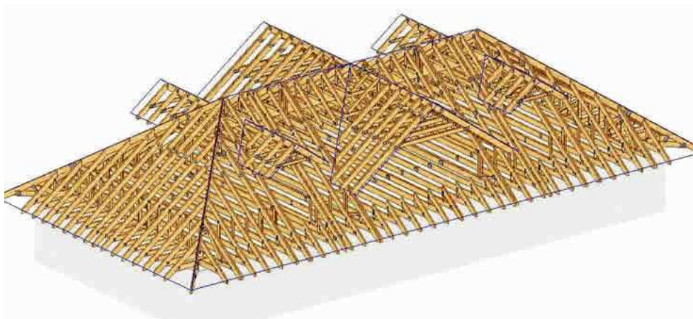
Rys. 6. Poddasze użytkowe z sześcioma lukarnami zaprojektowane w technologii kratownicowych więzarów drewnianych [7]
