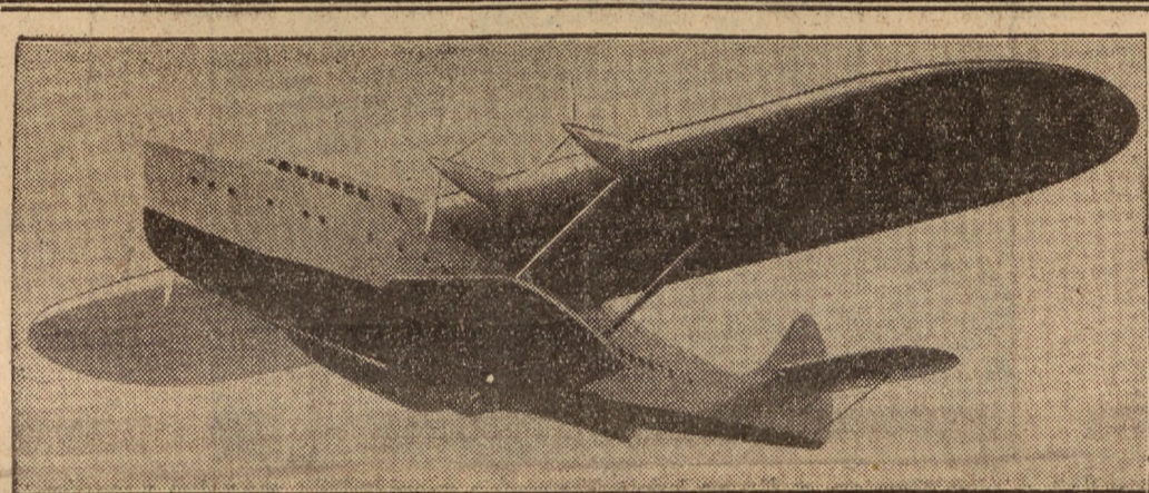
Na wystawie samolotowej w Sztokholmie zademonstrowano nowy typ samolotu, wytworzonego przez zakłady samolotowe Dornier. Samolot ten zaopatrzony jest w 8 motorów Diesla o sile 800—1000 H. P. każdy. Rozwinać może w nieprzerwanym locie na trasie 4 do 5 tysięcy kilometrów szybkość 250—300 km. na godzinę.
