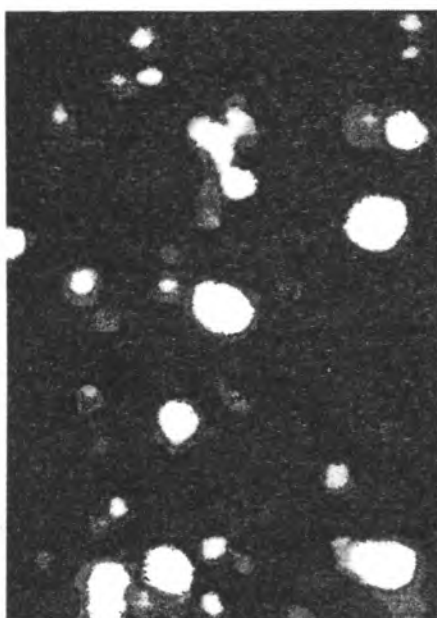
OBSERWACJE NAZIEMNE — HORYZONT W ODLEGŁOŚCI 7-8 mld ls.
