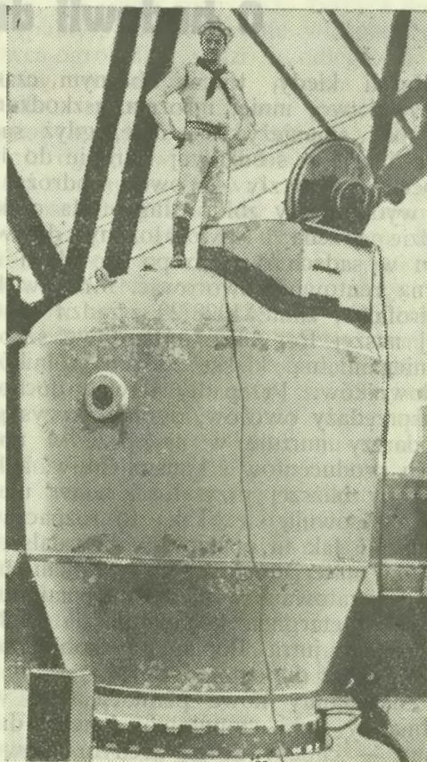
Przyrząd do ratowania załogi zatoniętych łodzi podwodnych
