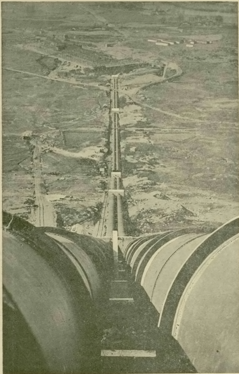
Pohled na elektrárnu a potrubí vodovodu u Fort William ve Skotsku.
