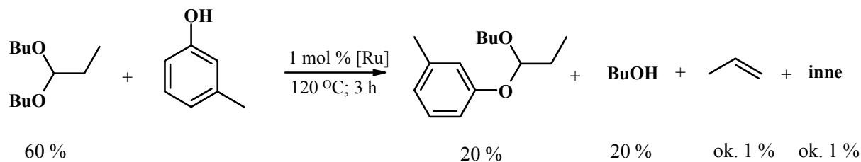
Schemat 61. Reakcja 1,1-dibutoksypropanu z m -krezolem w obecności [\text{RuCl}_2(\text{PPh}_3)_3]
