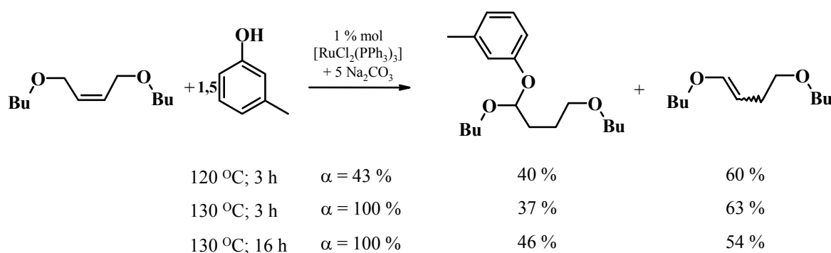
Schemat 46. Addycja m -krezolu do ( Z )-1,4-dibutoksy-2-buten (bez rozpuszczalnika).
