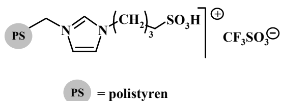
Rysunek 3. Immobilizowana na polistyrenie kwaśna ciecz jonowa [59].
