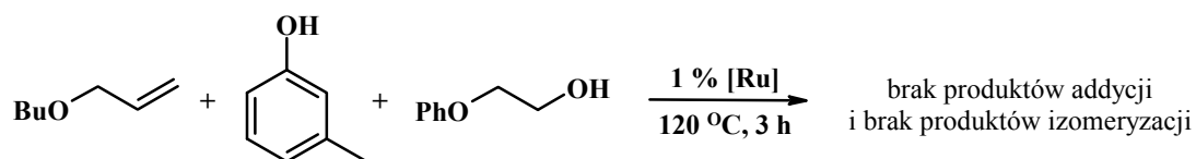
Schemat 50. Reakcja eteru allilowo-butyłowego z równomolową mieszaniną m -krezolu i 2-fenoksyetanolu. Warunki reakcji: 120\text{ }^\circ\text{C} , 3 h, bez rozpuszczalnika. Eter allilowy : m -krezol : 2-fenoksyetanol : [\text{RuCl}_2(\text{PPh}_3)_3] : \text{Na}_2\text{CO}_3 = 100 : 100 : 100 : 1 : 5. Brak produktów addycji i izomeryzacji.
