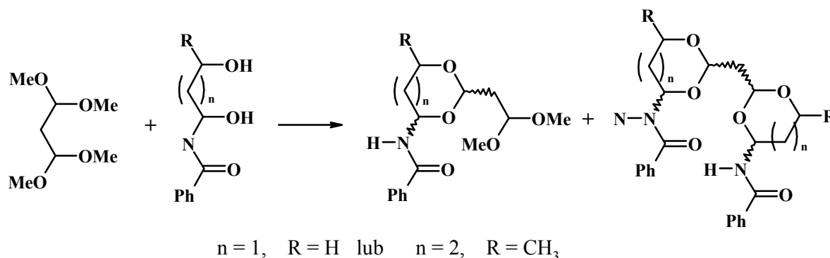
Schemat 7. Stereoselektywna transacetalizacja 1,1,3,3-tetrametoksypropanu w reakcji z różnymi N -benzyloaminodiolami prowadząca do pochodnych 1,3-dioksanu i 1,3-dioksepanu [10].
