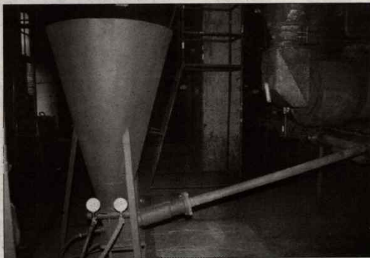
Pracownicy EC sami wykonali instalację podawania mialu drewnego do kotła
