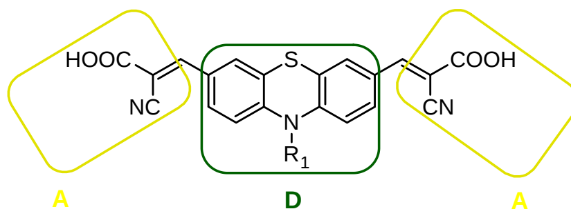
Rys. 32 Symetryczne pochodne kwasu dycyjanooctowego zawierające cząsteczkę N-alkilofenotiazyny, gdzie R_1 = C_2H_5, C_4H_9, C_8H_{17}, C_{12}H_{25} .
