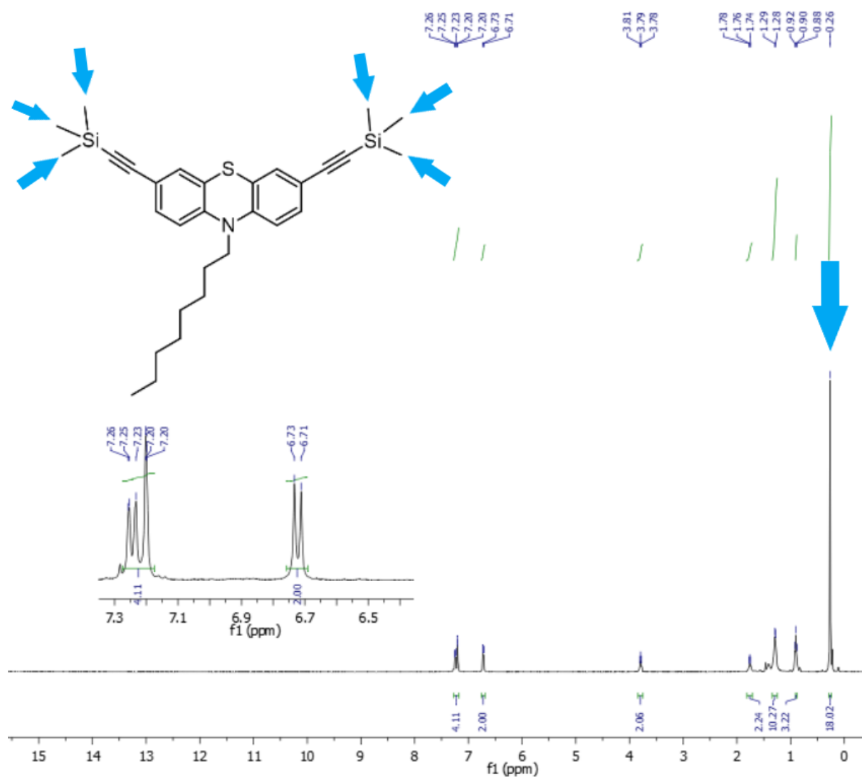
Rys. 39 Widmo ^1\text{H} NMR 3,7-bis(trimetylosililoetynylo)-10-oktylo-10 H -fenotiazyny ( 4b ).
