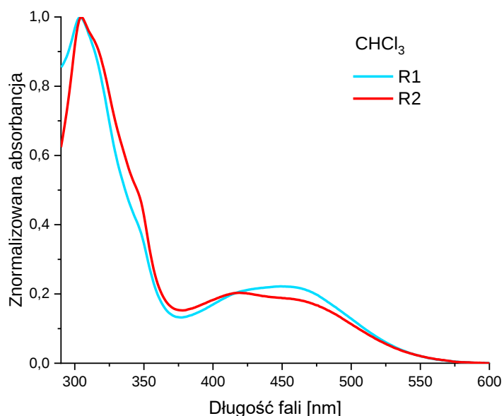
Rys. 78 Widma UV-Vis związków R1 oraz R2 w chloroformie ( c=10^{-5} \text{ mol}\cdot\text{L}^{-1} ).
