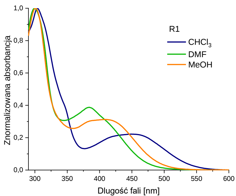
Rys. 79 Widma UV-Vis związku R1 zmierzone w \text{CHCl}_3 , DMF, MeOH ( c=10^{-5} \text{ mol}\cdot\text{L}^{-1} ).
