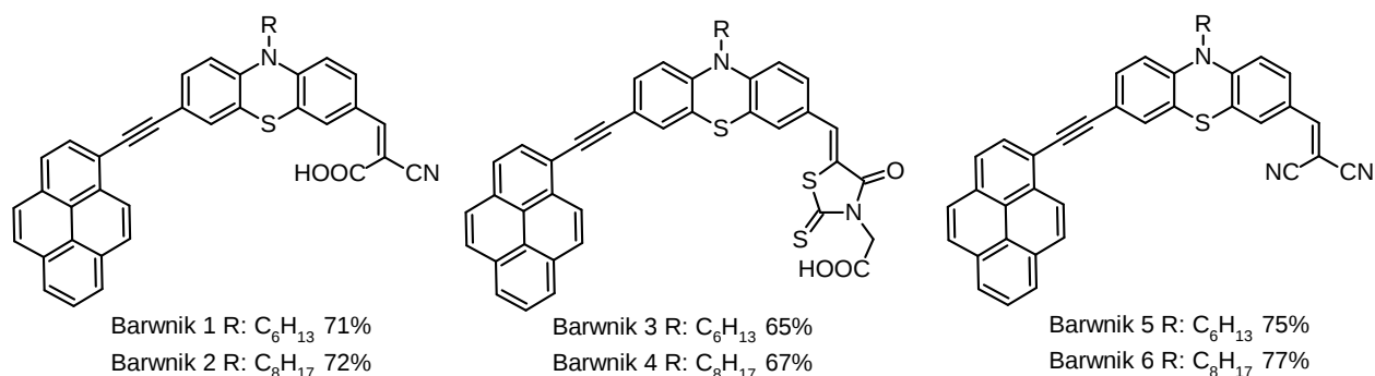
Rys. 28 Pirenowe, etynylowe pochodne fenotiazyny różniące się grupami elektronoakceptorowymi oraz długością łańcucha alkilowego [99].
