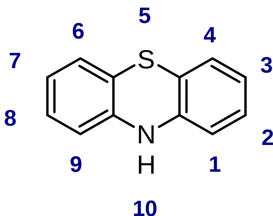
Rys. 5 Struktura cząsteczki 10 H -fentiazyny wraz z numeracją pozycji w pierścieniu.
