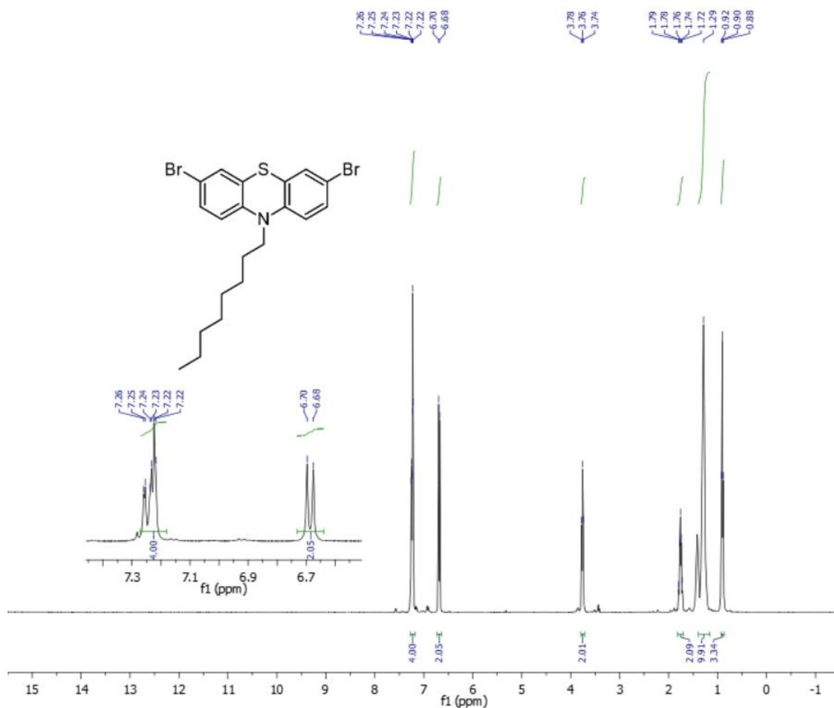
Rys. 38 Widmo 1 H NMR 3,7-dibromo-10-oktylo-10 H -fenotiazyny ( 2c ).
