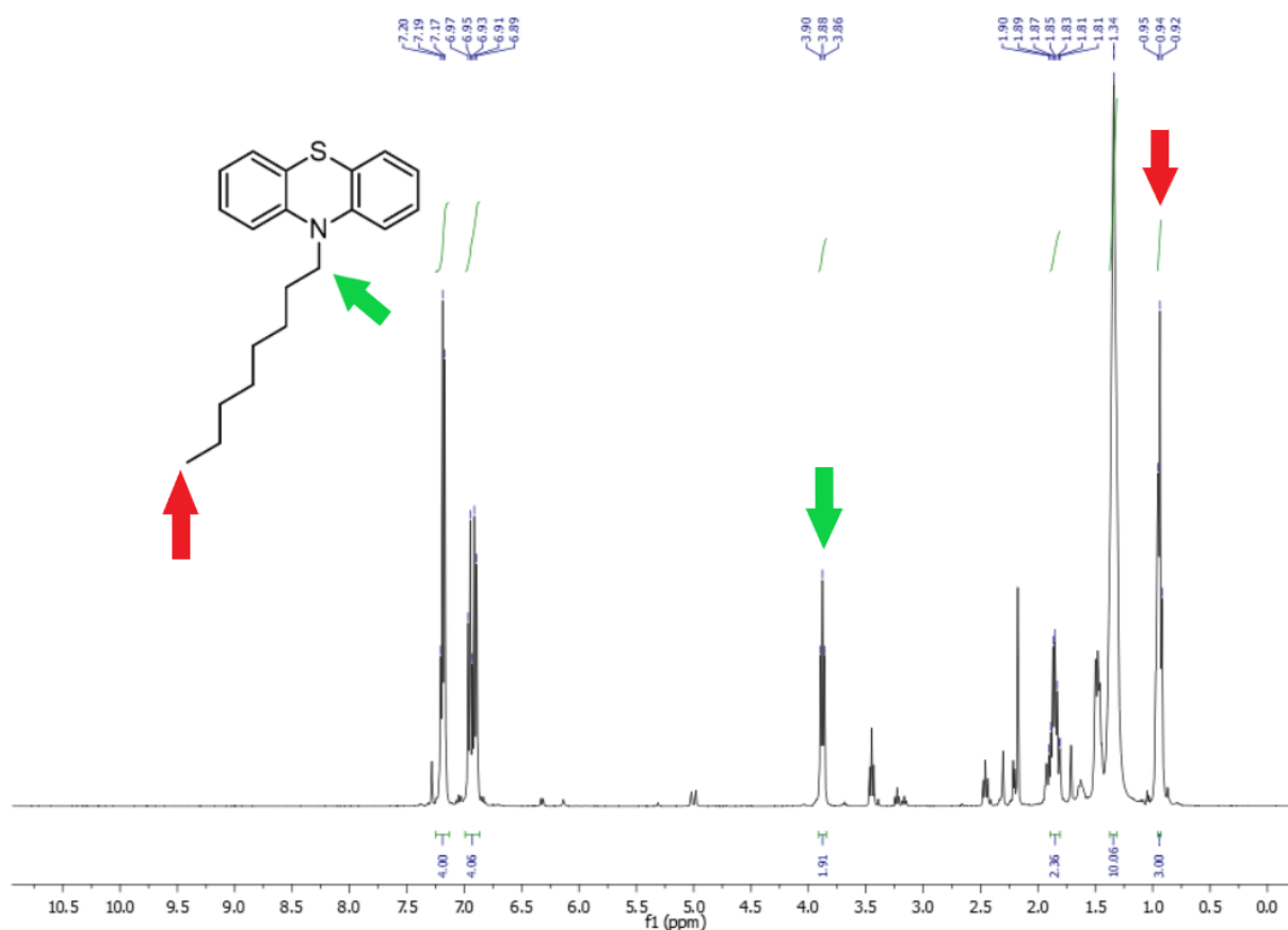
Rys. 37 Widmo ^1\text{H} NMR 10-oktylo-10 H -fenotiazyny ( 1c ).
