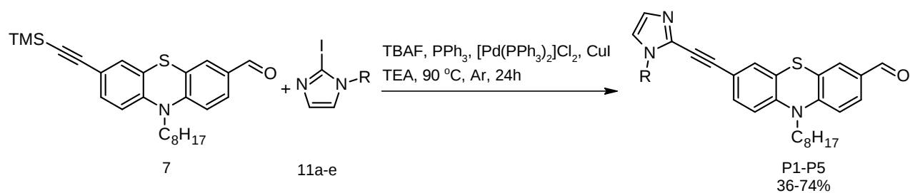
Rys. 66 Schemat syntezy niesymetrycznych, etynyłowych pochodnych N-oktylofenotiazyny z podstawnikami N-alkiloimidazolyłowymi ( P1-P5 ).
