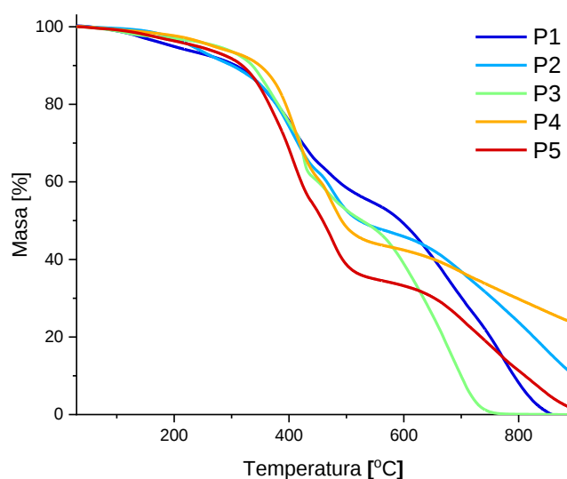
Rys. 69 Krzywe TGA związków P1-P5 .
