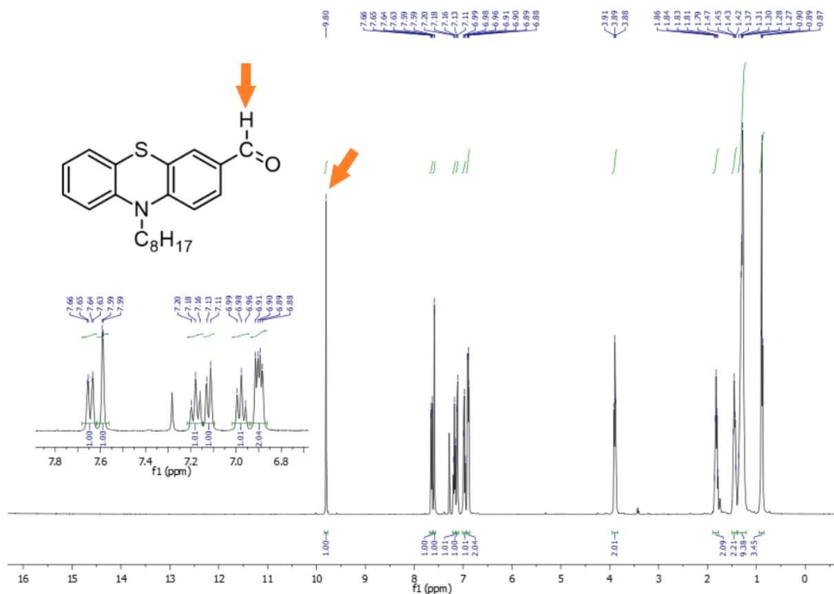
Rys. 61 Widmo ^1\text{H} NMR 10-oktylo-10H-fenotiazyno-3-karboaldehydu (5).
