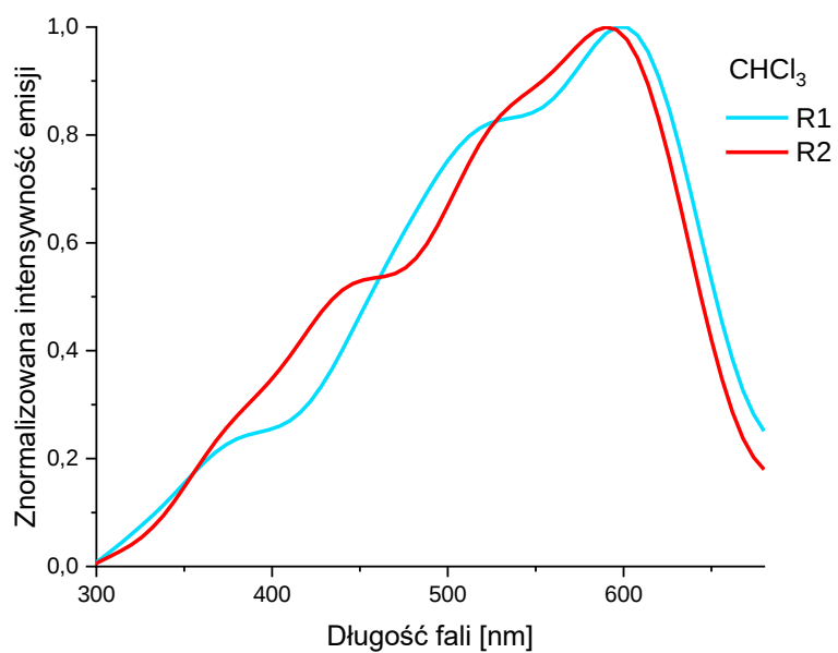
Rys. 81 Widma emisyjne związków R1 oraz R2 w chloroformie ( c=10^{-5} \text{ mol}\cdot\text{L}^{-1} ).
