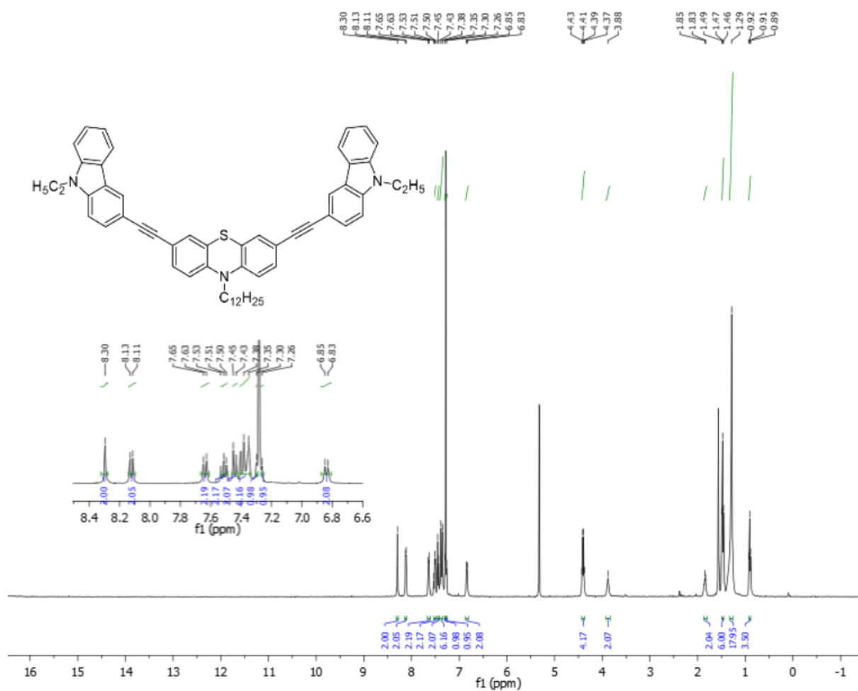
Rys. 44 Widmo 1 H NMR 3,7-bis((N-etylokarbaz-3-ylo)etynylo)-N-dodecylofenotiazyny ( PTZ-O ).
