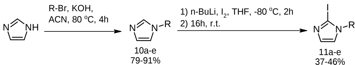
Rys. 63 Schemat otrzymywania serii 1-jodo-N-alkilimidazoli ( 11a-e ), gdzie R to łańcuch C 4 H 9 , C 6 H 13 , C 10 H 21 , C 12 H 25 lub C 16 H 33 .
