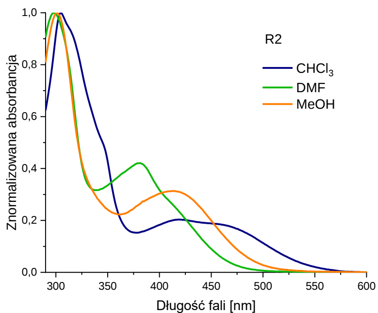
Rys. 80 Widma UV-Vis związku R2 zmierzone w \text{CHCl}_3 , DMF, MeOH ( c=10^{-5} \text{ mol}\cdot\text{L}^{-1} ).
