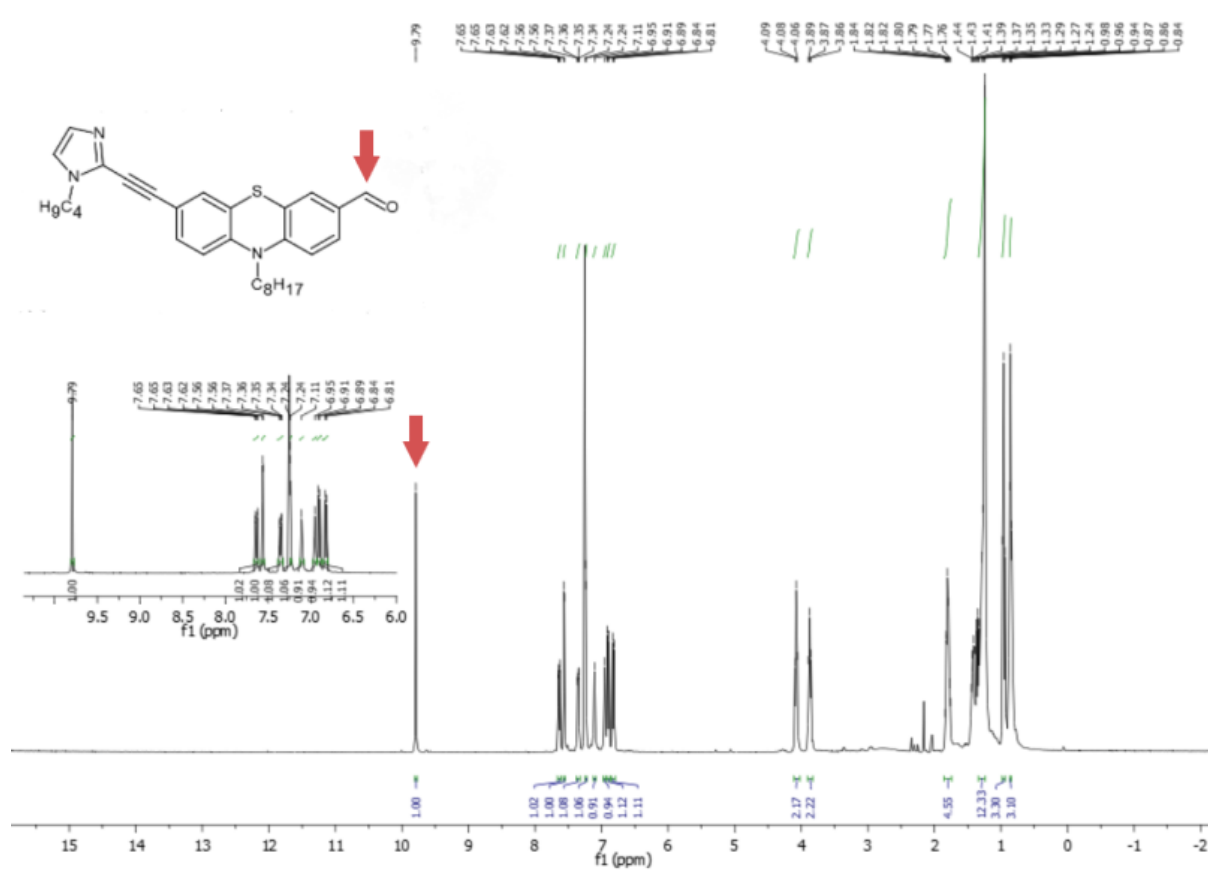
Rys. 67 Widmo ^1\text{H} NMR 7-[2-(1-butylo-1 H -imidazolylo)etynylo]-10-oktylo-10 H -fenotiazyno-3-karboaldehydu ( P1 ).
