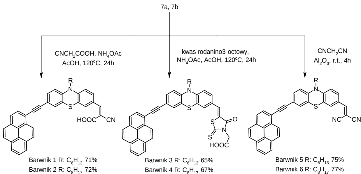
Rys. 20 Otrzymywanie barwników 1-6, z różnymi grupami elektronoakceptorowymi [99].
