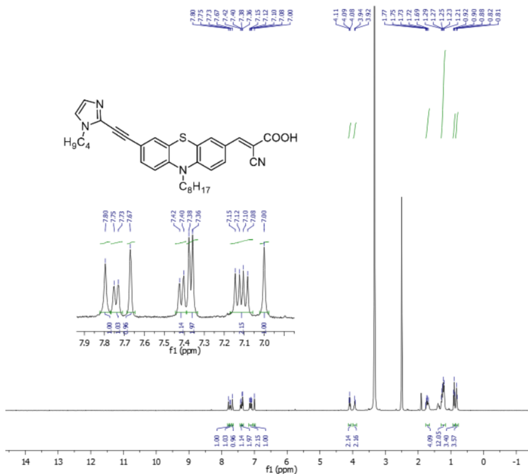
Rys. 76 Widmo ^1\text{H} NMR pochodnej R1 .
