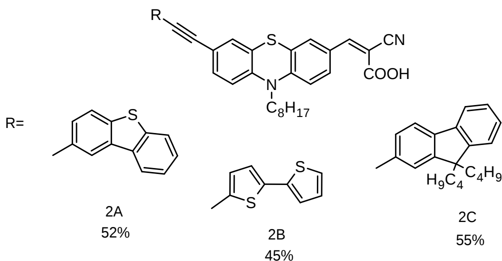
Rys. 23 Pochodne fenotiazyny o układzie D- \pi -D- \pi -A z podstawnikami dibenzotiofenylowym (2A), 2,2'-bitienylowym (2B) i 9,9'-dibutyłfluorenylowym (2C) oraz elektronoakceptorową grupą cyjanooctową [101].
