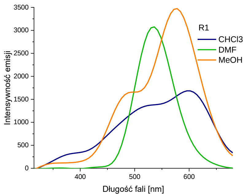
Rys. 82 Widma emisyjne związku R1 zmierzone w \text{CHCl}_3 , DMF, MeOH ( c=10^{-5} \text{ mol}\cdot\text{L}^{-1} ).
