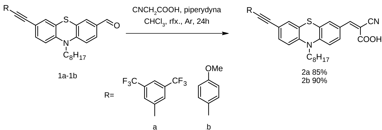
Rys. 22 Schemat syntezy oraz struktury pochodnych 2a oraz 2b o układzie A/D- \pi -D- \pi -A [100].
