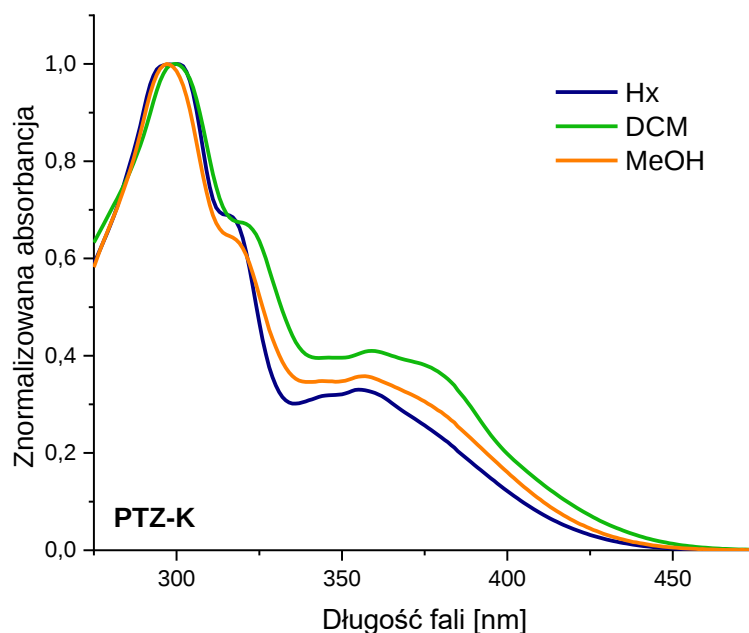
Rys 50 Widma UV-Vis związku PTZ-K zmierzone w Hx, DCM oraz MeOH ( c=10^{-5} \text{ mol} \cdot \text{L}^{-1} ).
