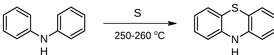
Rys. 1 Schemat pierwszej syntezy 10 H -fenotiazyny przeprowadzonej przez Berenthseana [7].
