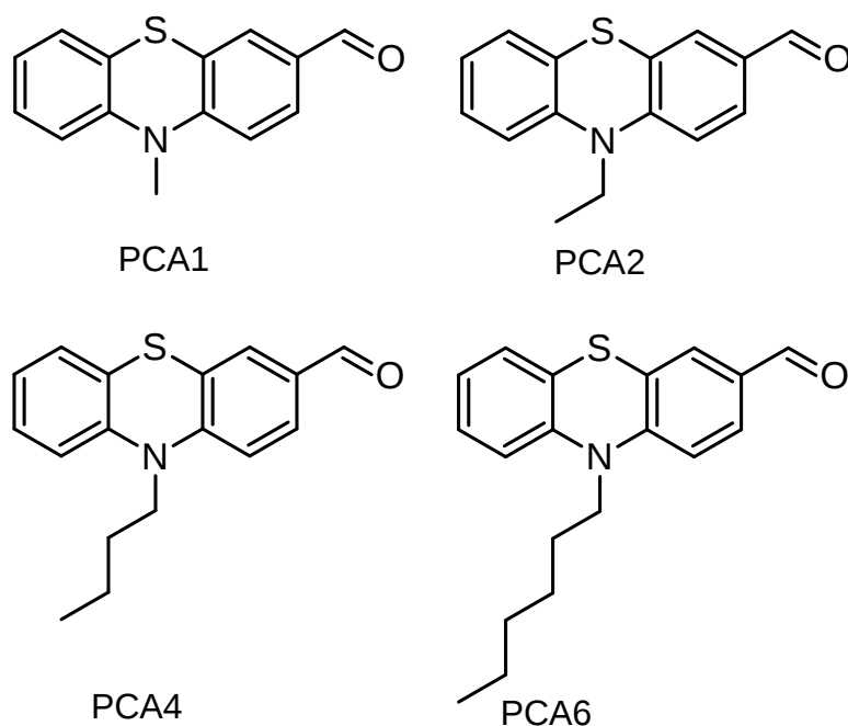
Rys. 27 Struktury PCA1, PCA2, PCA4, PCA6 z łańcuchami alkilowymi metylowym, etylowym, butylowym oraz heksylowym [81].
