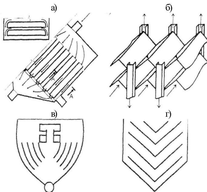
Рис. 4. Форма полиць поличкових тонкошарових відстійників а – П-подібні, б – хвилеподібні, в – криволінійні, г – V-подібні
