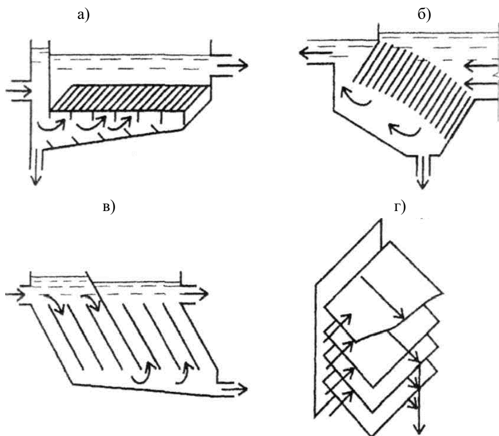
Рис. 5. Поличкові тонкошарові відстійники а – з поздовжнім зворотним нахилом полиць; б – з поздовжнім прямим нахилом полиць; в – з поздовжнім комбінованим набором полиць; г – з поперечним нахилом полиць
