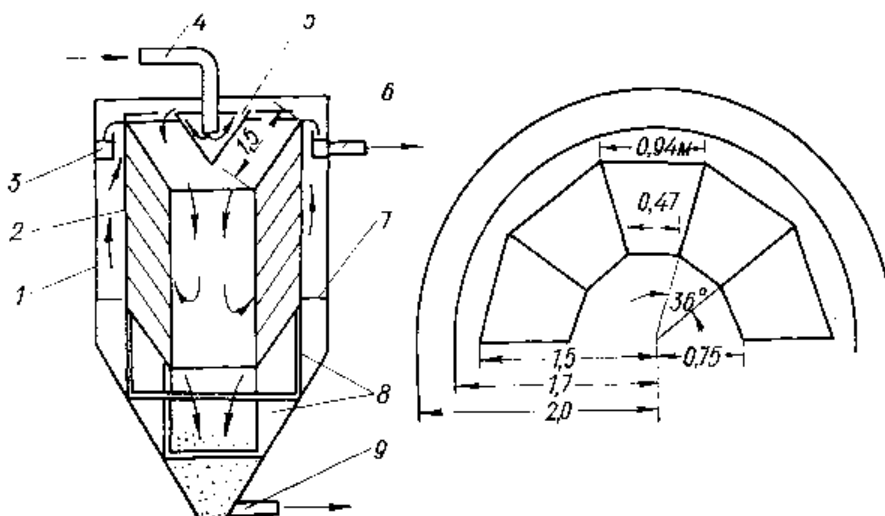
Рис. 2. Встановлення тонкошарових модулів у вертикальному відстійнику
