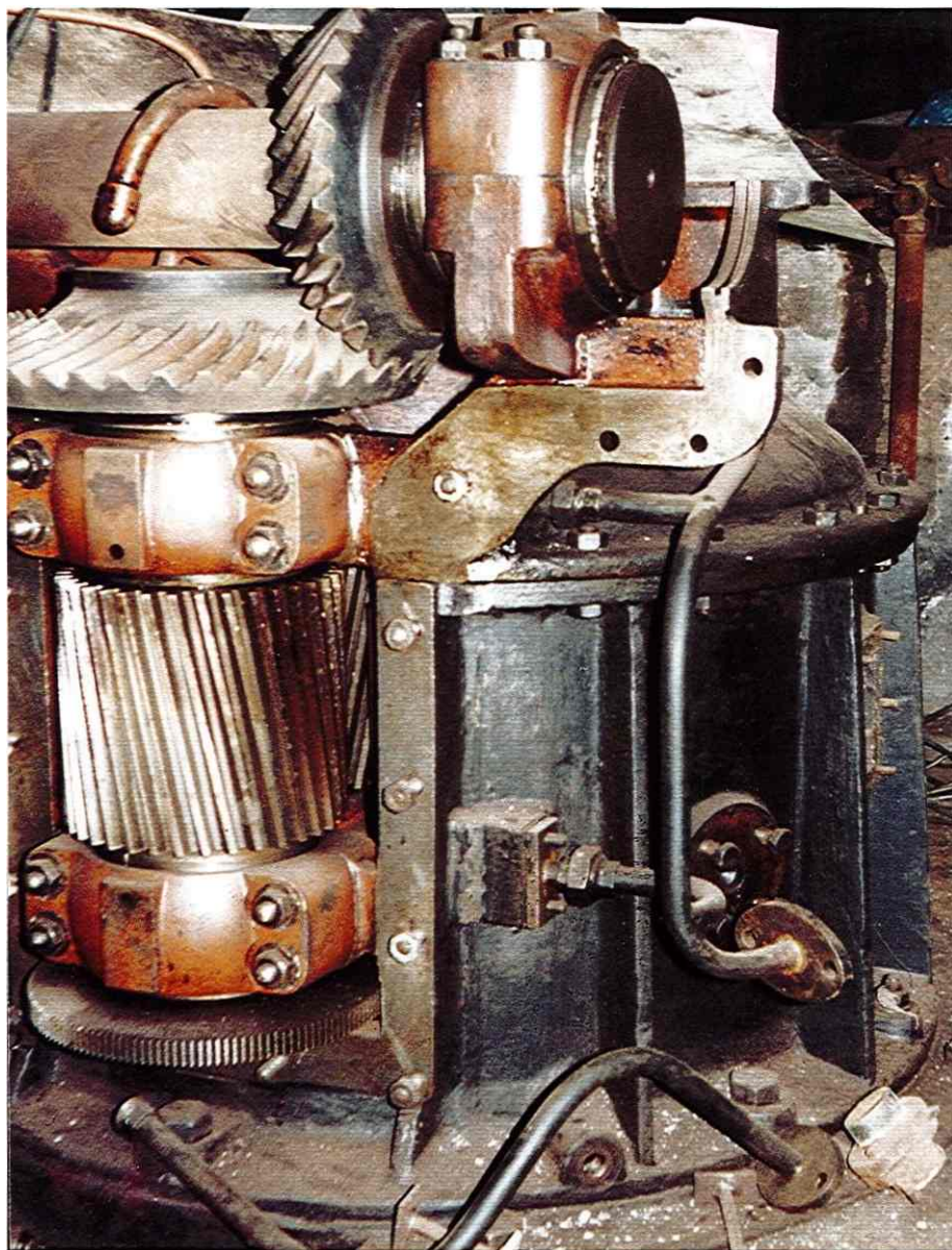
Diese Turbine, ein Produkt der Firma J. M. Voith aus Heidenheim, stammt aus den Anfängen der Krappitzer Stromversorgung.
