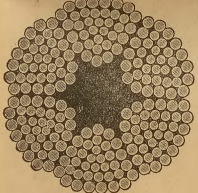
Querschnitt eines 3-Kant-Litzenseiles System Deichsel
