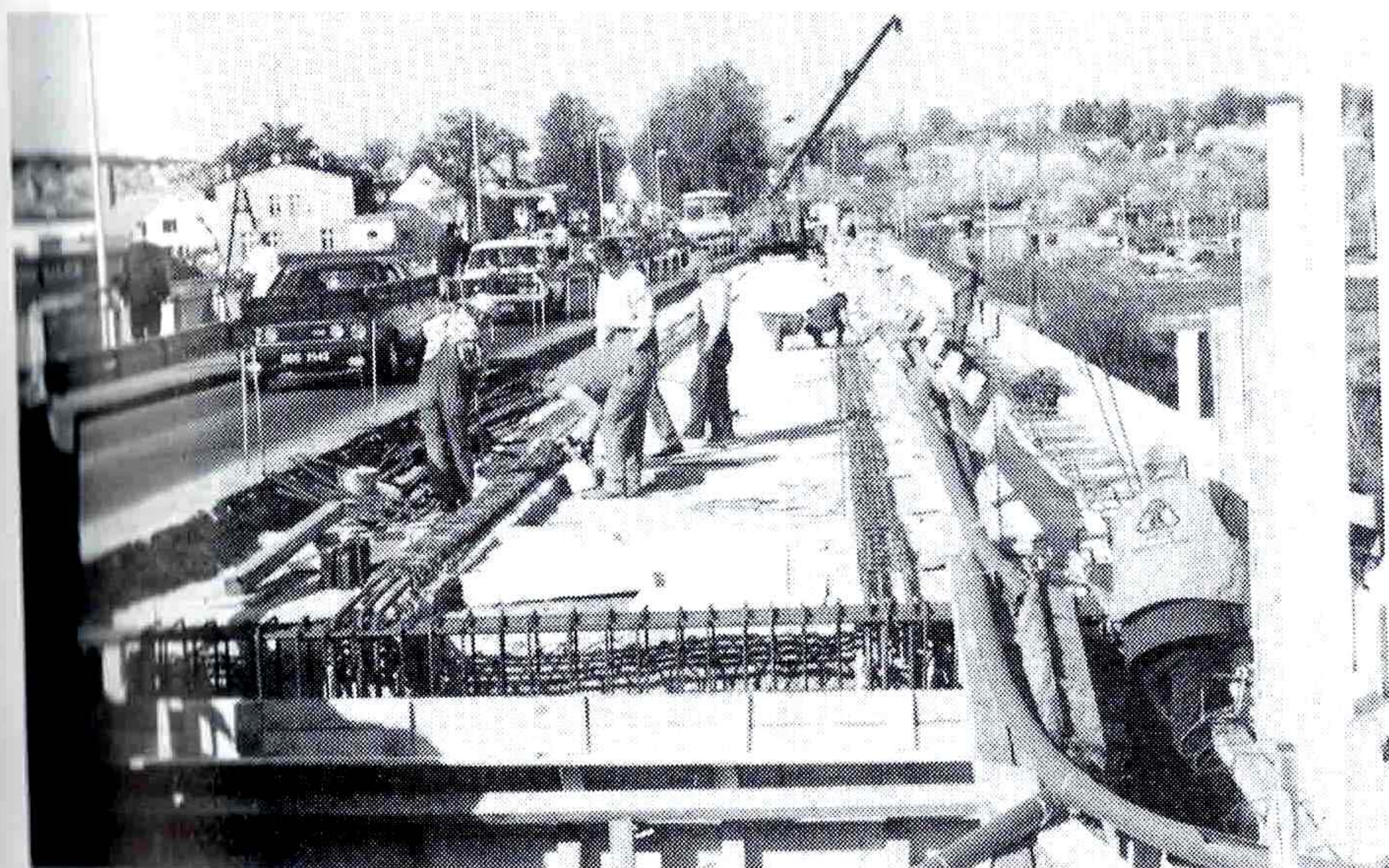
Verstärkung der Brückenkonstruktion
