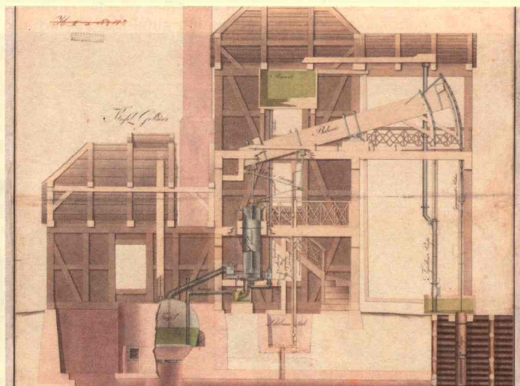
20 calowa maszyna parowa systemu Newcommena dla kopalni w Tarnowskich Górach, wykonana w całości w Królewskiej Hucie Małapanew w Ożimku w roku 1788 (Rysunek z archiwum Wyższego Urzędu Górniczego we Wrocławiu, w zbiorach Muzeum Górnictwa Węglowego w Zabrze).
