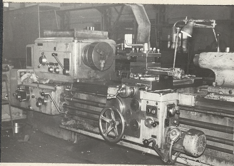
Tokarka do obróbki elementów maszyn i urządzeń górniczych
