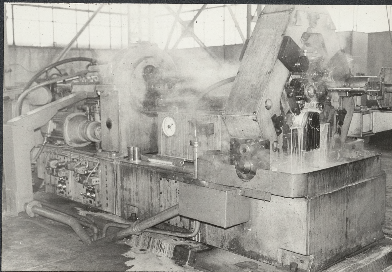
Linia automatyczna do produkcji rur ożebrowanych
