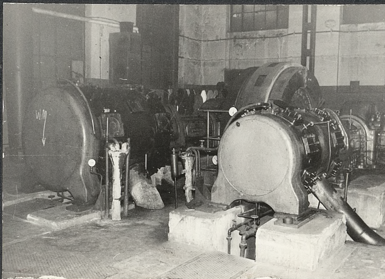
Kompresory typu 2WG stosowane do zasilania sieci sprężonego powietrza w kop. „Grzeł Biały”
