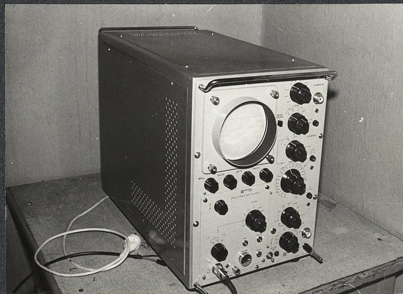
Lokalizator uszkodzeń kabli JKL-5 do pomiaru stanu izolacji i lokalizacji uszkodzeń kabli elektrycznych.
