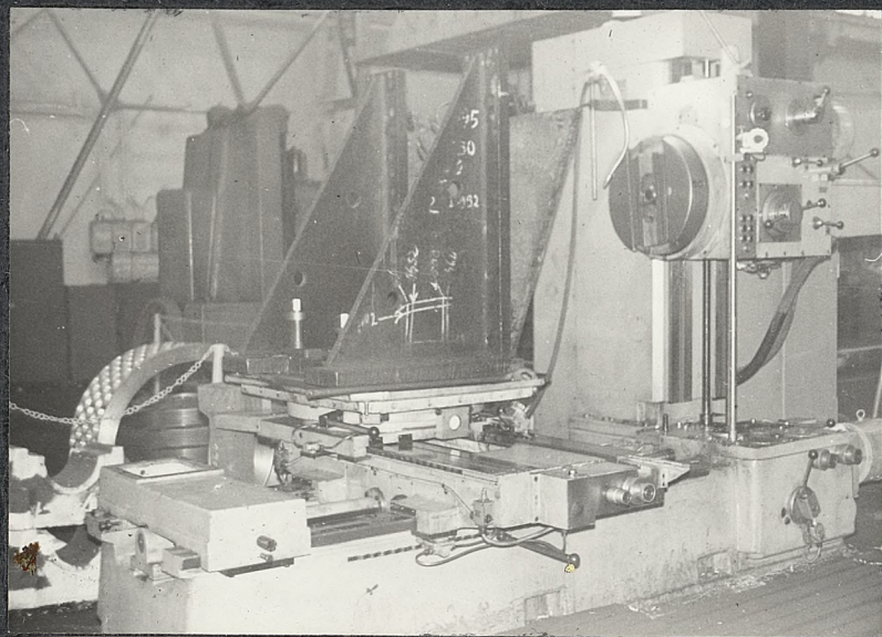
Wytaczarka - frezarka do obróbki dużych elementów
