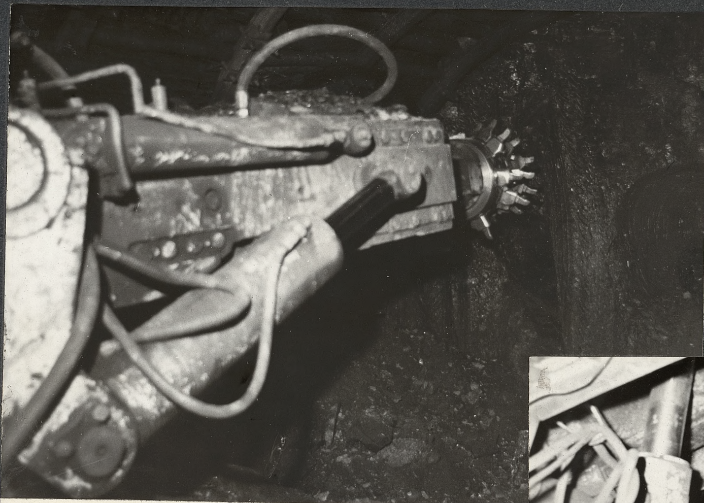
Kombajn chodnikowy PK-9r do drażnienia wyrobisk chodnikowych przygotowanych
