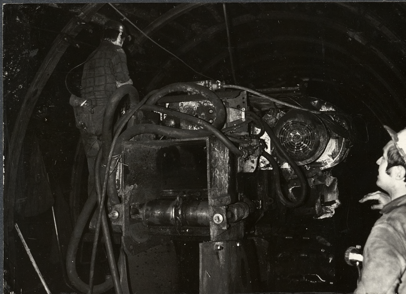
Kombajn chodnikowy PK-9r przeznaczony do szyb- kościowego drażenia wyrobisk przygotawawczych
