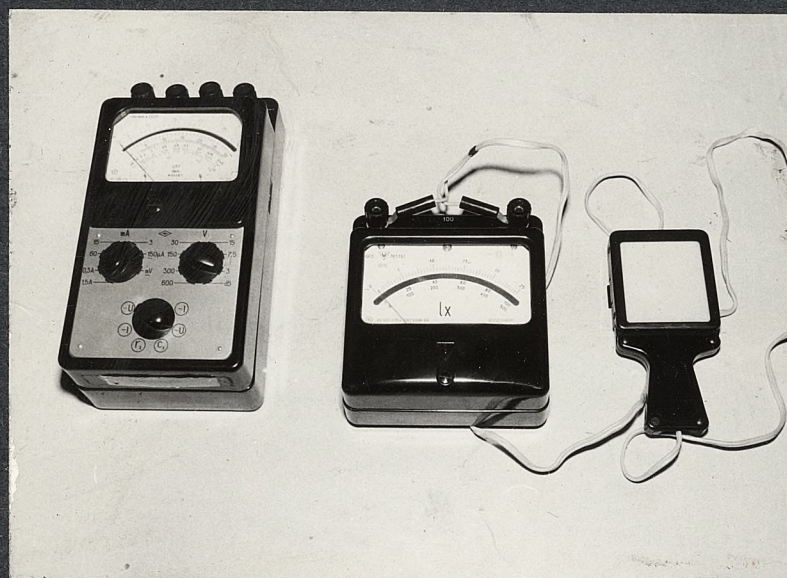
Aparatura kontrolno-pomiarowa do pomiaru natężenia oświetlenia i pomiaru prądu w urządzeniach elektrycznych.
