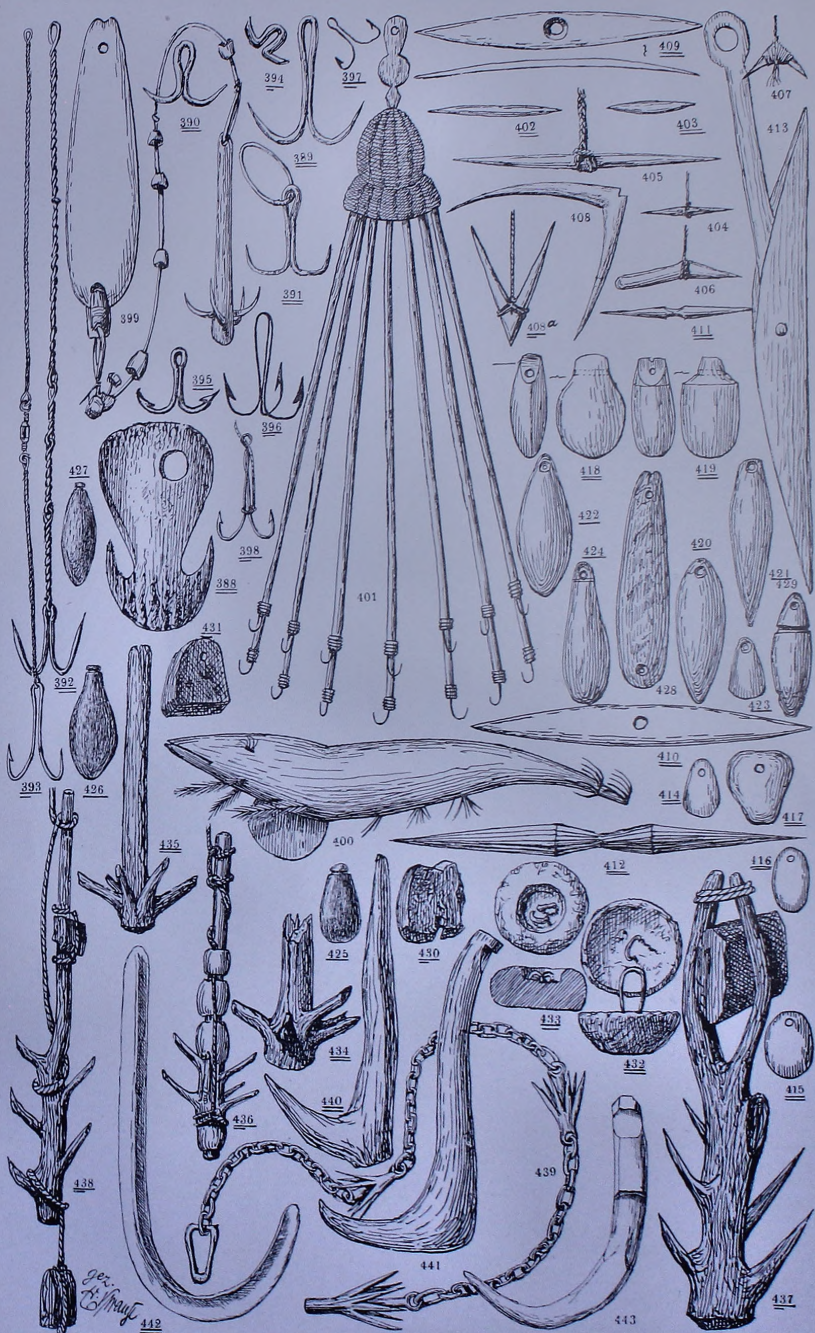
Eduard Krause. Vorgeschichtliche Fischereigeräte und neuere Vergleichsstücke. X. Bezeichnung: 1 Europa, vorgeschichtlich; 1 Europa, später; 1 ausser Europa, vor- geschichtlich; 1 ausser Europa, später.
