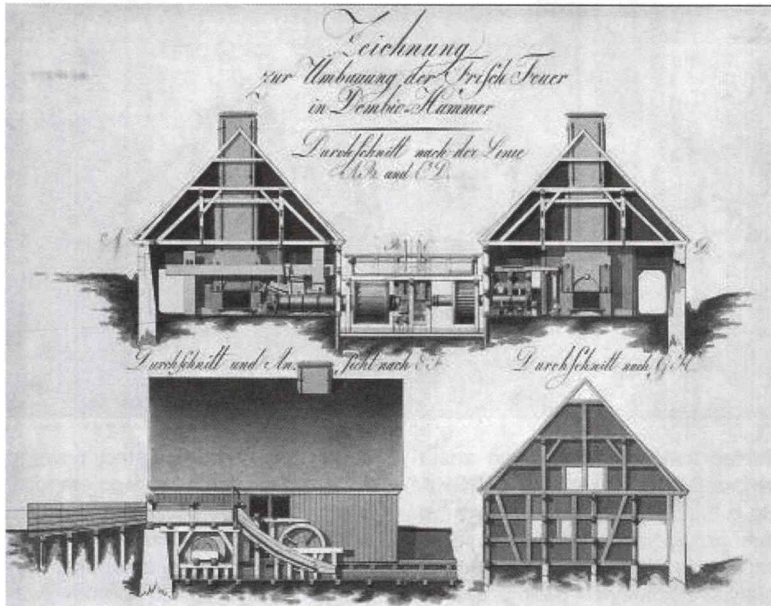
Budynki huty w Dębskiej Kuźni, po ich modernizacji w początkach XIX wieku, na rysunku ze zbiorów Wyższego Urzędu Górniczego we Wrocławiu, przechowywanym w Muzeum Górnictwa Węglowego w Zabrze.
