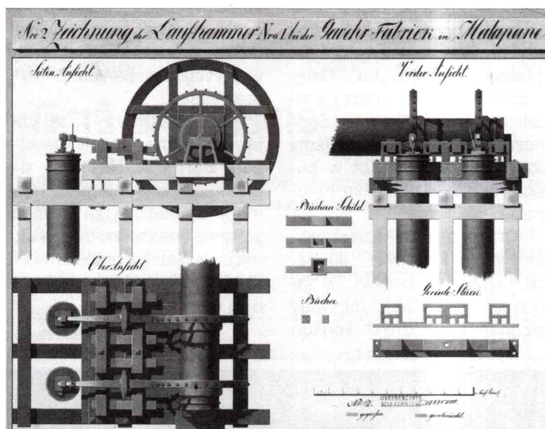
Młoty napędzane kołem wodnym w fabryce armatur huty w Ozimku. Rycina z roku 1820 ze zbiorów Muzeum Górnictwa Węglowego w Zabrzu.
