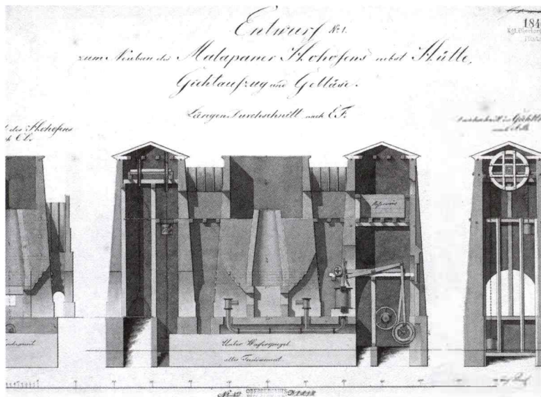
Urządzenia wysokiego pieca huty w Ozimku po modernizacji na początku XIX wieku. Rycina ze zbiorów Muzeum Górnictwa Węglowego w Zabrzu.
